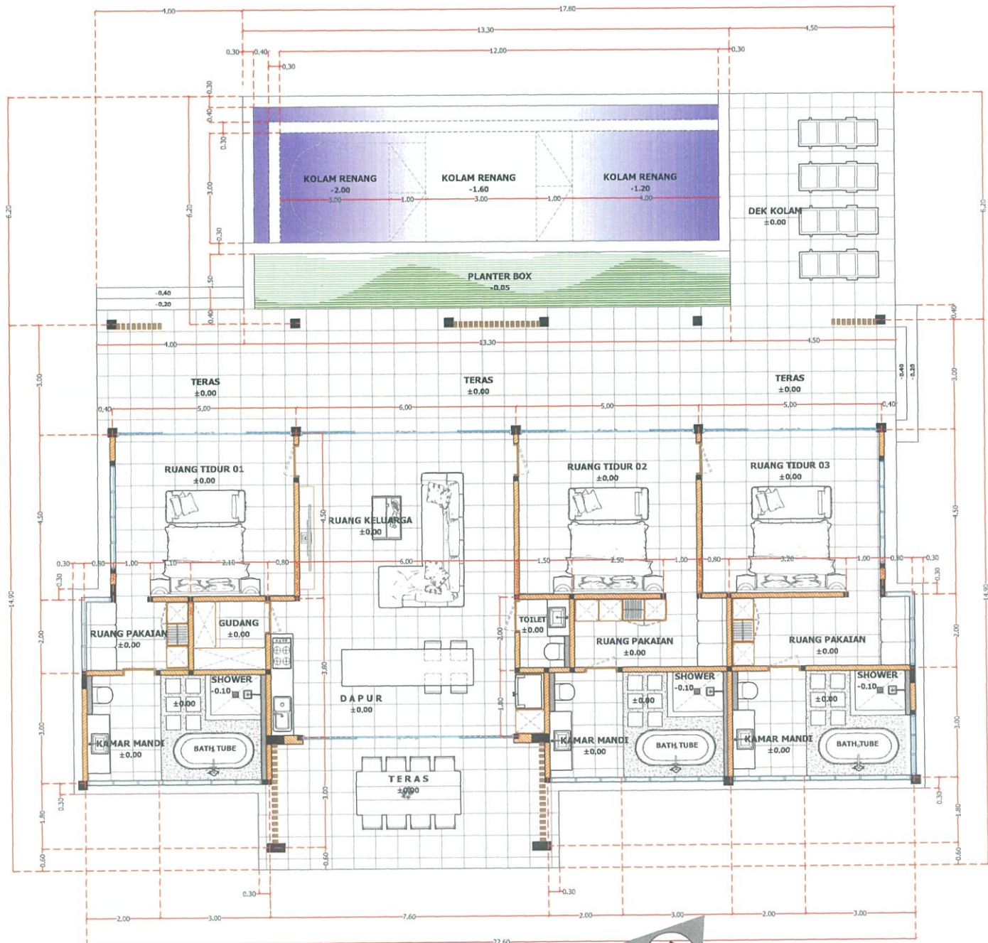
DENAH RUMAH scale 1: 100
