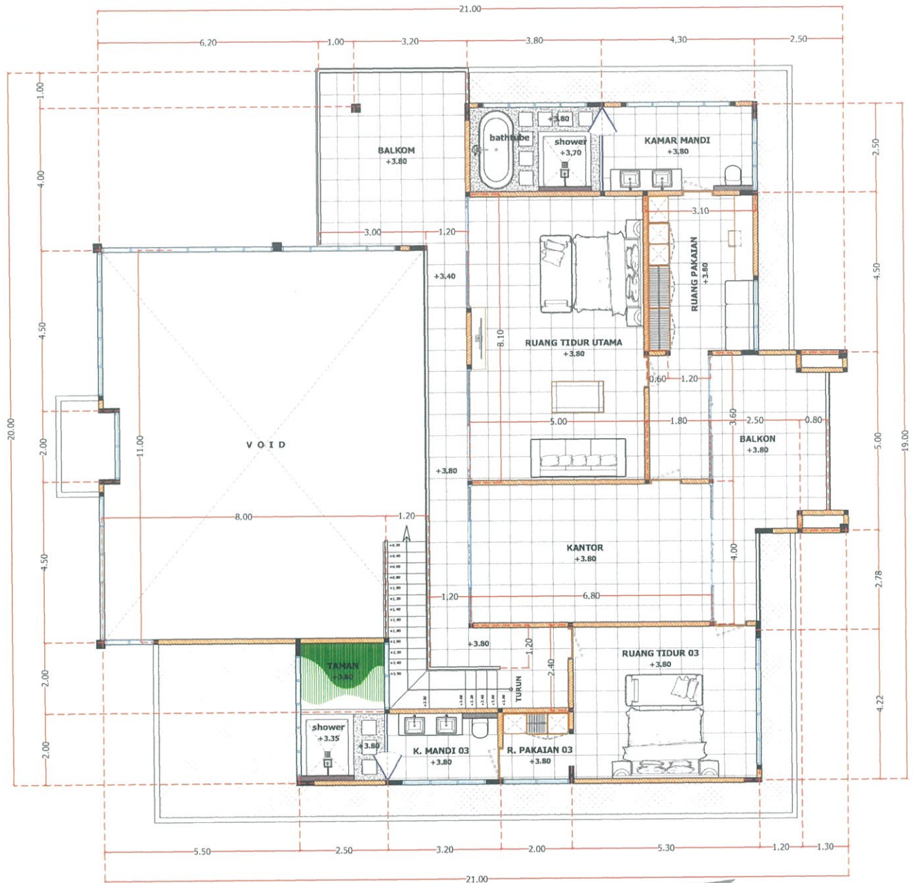
RUMAH UTAMA - DENAH LANTAI 02
